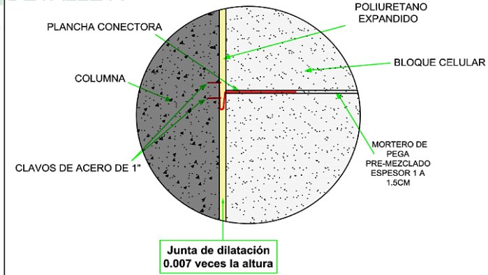
DETALLE A
