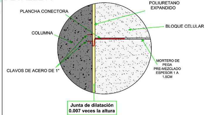
DETALLE A
