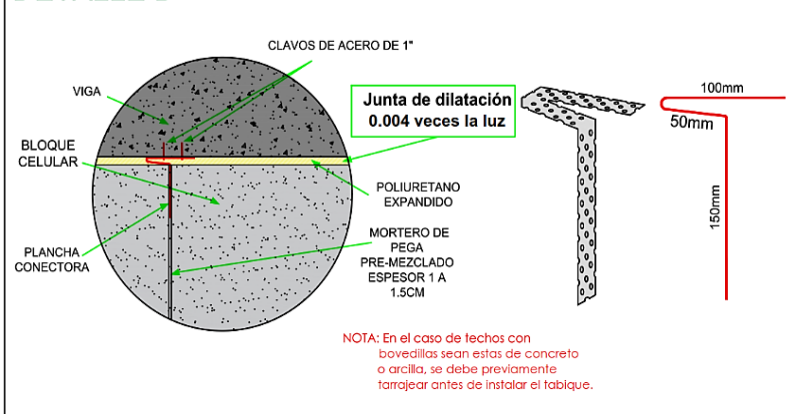
DETALLE B
